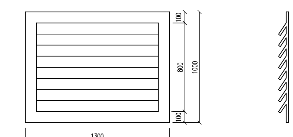
PART. GRIGLIATO ZINCATO A LAMELLE ORIZZONTALI
